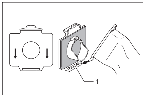
► 1. Rainure inférieure
