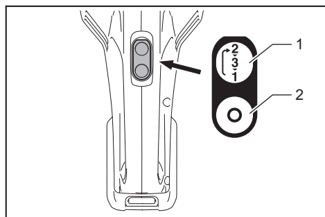
► 1. Bouton MARCHE/changement de vitesse 2. Bouton ARRÊT
