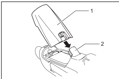
► 1. Couvercle avant 2. Raccord de couvercle avant
